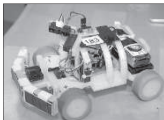
Робот, сконструированный Матисом Буксом.
