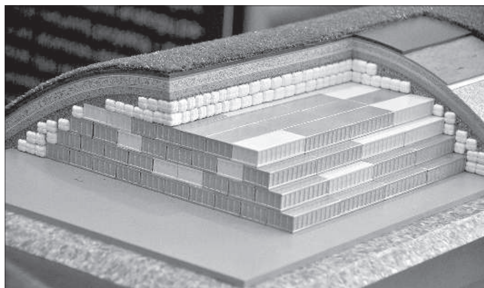
Макет хранилища радиоактивных отходов.
