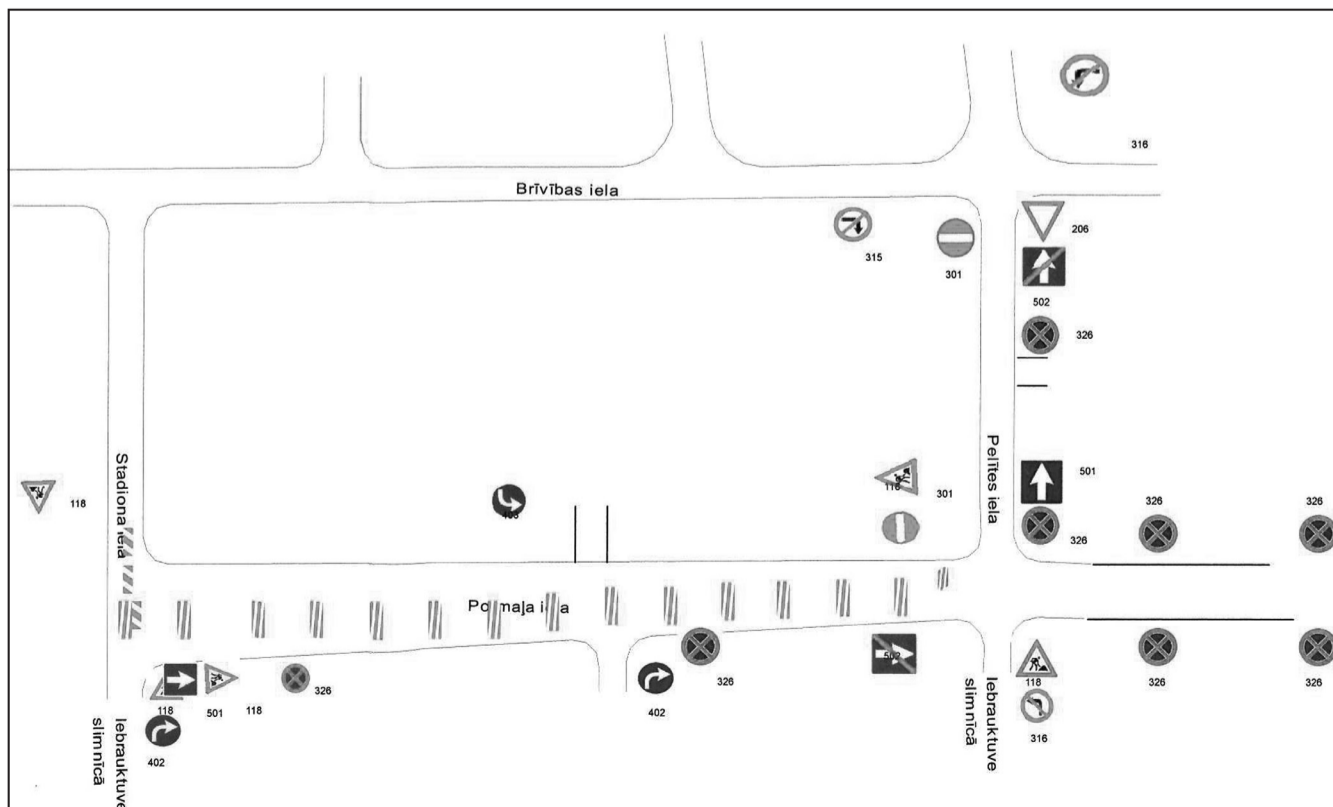
Satiksmes organizācijas shēma projekta „Satiksmes drošības uzlabošana pie Jēkabpils rajona centrālās slimnīcas un poliklinikas” būvniecības darbu laikā
