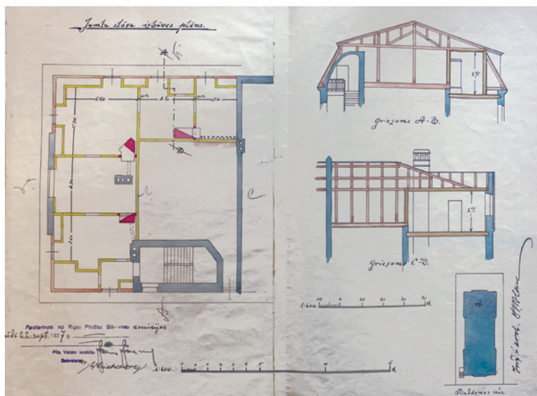
10. attēls. Arhitekta H. Blaua izstrādātais nama Baldones ielā 11 jumta stāva izbūves projekts (1927).
