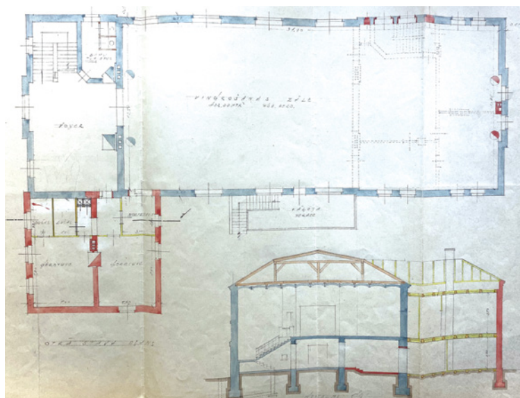
13. attēls. Arhitekta A. Laukirbes ĀVSB nama vingrošanas zāles otrā stāva pārbūves un ēkas piebūves plāns (1936).
