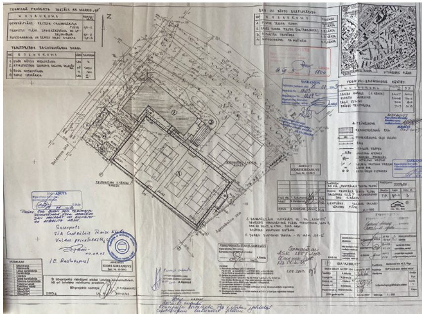
22. attēls. Teritorijas plānojums Baldones ielā 7 (2003).
