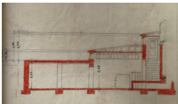
16. attēls. Katla telpas Baldones ielā 7 plāns un griezums (1949).
