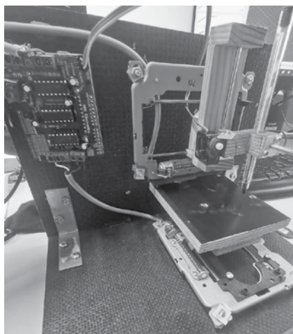
Rodrigo uzbūvētais CNC miniprinteris.
