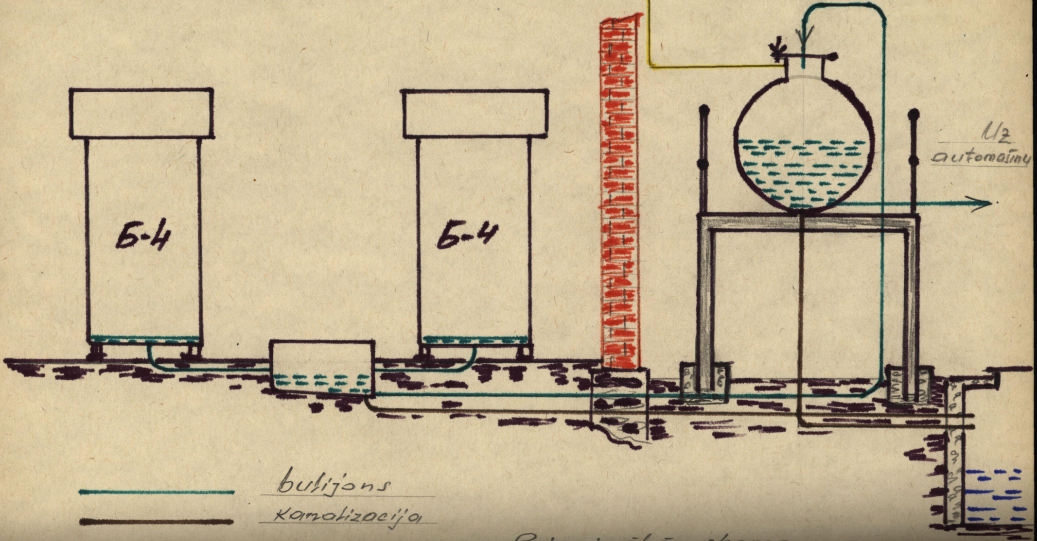
Principālā shema bulijona saistīšanai
