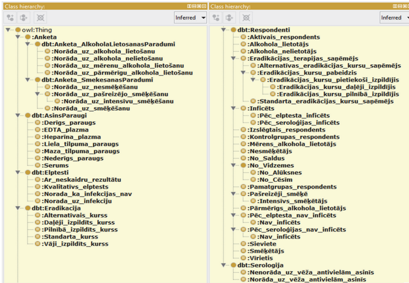
Fig. 4. IRDIS ontology.
