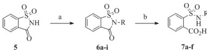
7. att. Saharīna atvasinājumu sintēze.
