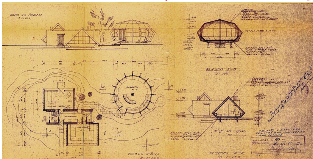
MĀJU SKICE. Postažu ģimenes vasarnicas Zvejniekiemā projekta (1971. g.) lapa. Kopija. Foto: no P. Postaža personiskā arhīva.
