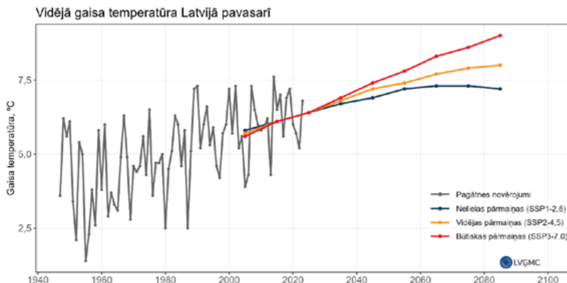
18. attēls Vidējā gaisa temperatūra Latvijā pavasarī kopš 1947. gada (novērojumu dati) līdz 2100. gadam (klimata pārmaiņu modeļu scenāriju SSP1 2,6; SSP2-4,5 un SSP3-7,0 dati)
