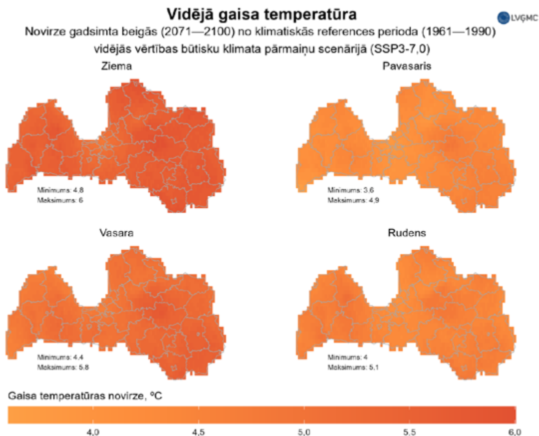
14. attēls Vidējās gaisa temperatūras pieaugums ziemā, pavasarī, vasarā un rudenī, salīdzinot klimata pārmaiņu modeļu prognozētās 2071. līdz 2100. gada vērtības (SSP3-7,0) ar klimatiskās references periodā (1961.–1990. gads) novērotajām vērtībām
