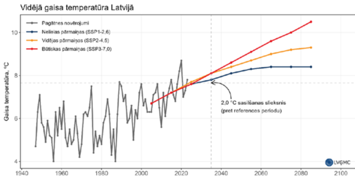
7. attēls Latvijas vidējā gaisa temperatūra kopš 1947. gada (novērojumu dati) līdz 2100. gadam (klimata pārmaiņu modeļu scenāriju SSP1-2,6; SSP2-4,5 un SSP3-7,0 dati)
