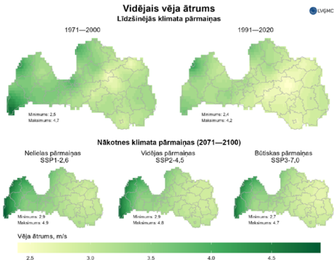
37. attēls Augšējā rindā: Vidējais vēja ātrums Latvijā no 1971. līdz 2010. gadam un klimatiskās normas periodā (1991.–2020. gads), kas balstīts uz LVĢMC meteoroloģisko novērojumu staciju datiem. Apakšējā rindā: Vidējais vēja ātrums Latvijā, kas 21. gadsimta beigām (2071.–2100. gads) aprēķināts balstoties uz klimata pārmaiņu modeļu scenārijiem SSP1-2,6; SSP2-4,5 un SSP3-7,0
