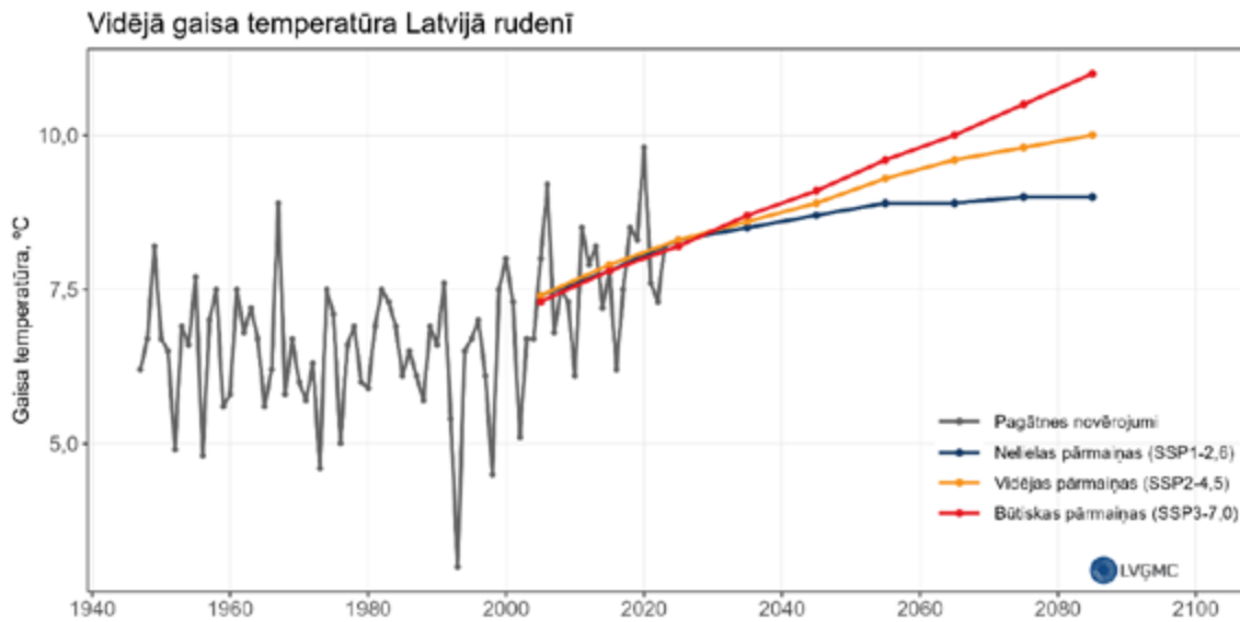
21. attēls Vidējā gaisa temperatūra Latvijā rudenī kopš 1947. gada (novērojumu dati) līdz 2100. gadam (klimata pārmaiņu modeļu scenāriju SSP1-2,6; SSP2-4,5 un SSP3-7,0 dati)
