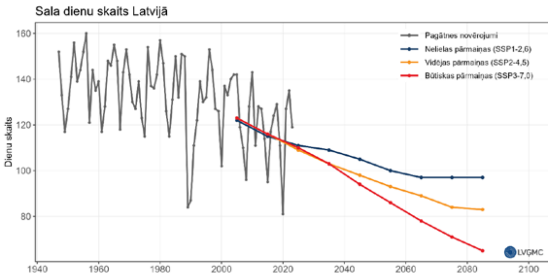
16. attēls Sala dienu skaits Latvijā kopš 1947. gada (novērojumu dati) līdz 2100. gadam (klimata pārmaiņu modeļu scenāriju SSP1-2,6; SSP2-4,5 un SSP3-7,0 dati)
