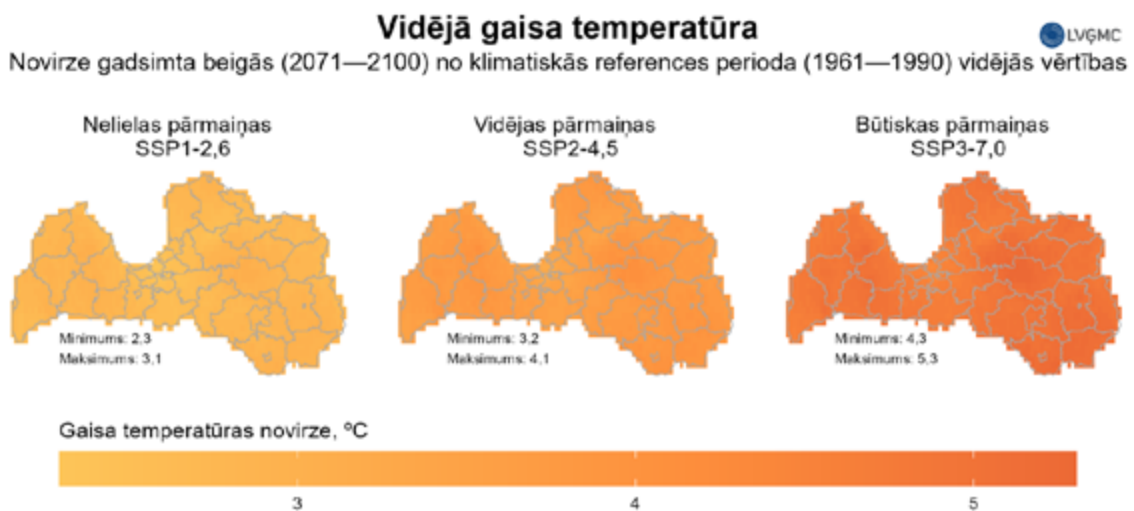
8. attēls Vidējās gaisa temperatūras pieaugums Latvijā 21. gadsimta beigās salīdzinājumā ar klimatiskās references perioda vērtībām
