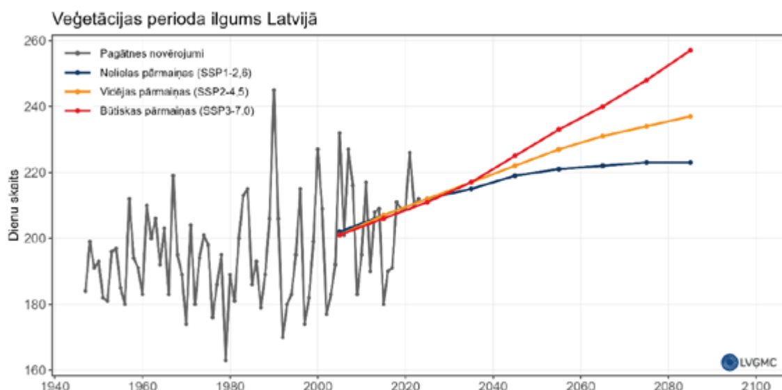
12. attēls Veģetācijas perioda ilgums Latvijā kopš 1947. gada (novērojumu dati) līdz 2100. gadam (klimata pārmaiņu modeļu scenāriju SSP1-2,6; SSP2-4,5 un SSP3-7,0 dati)
