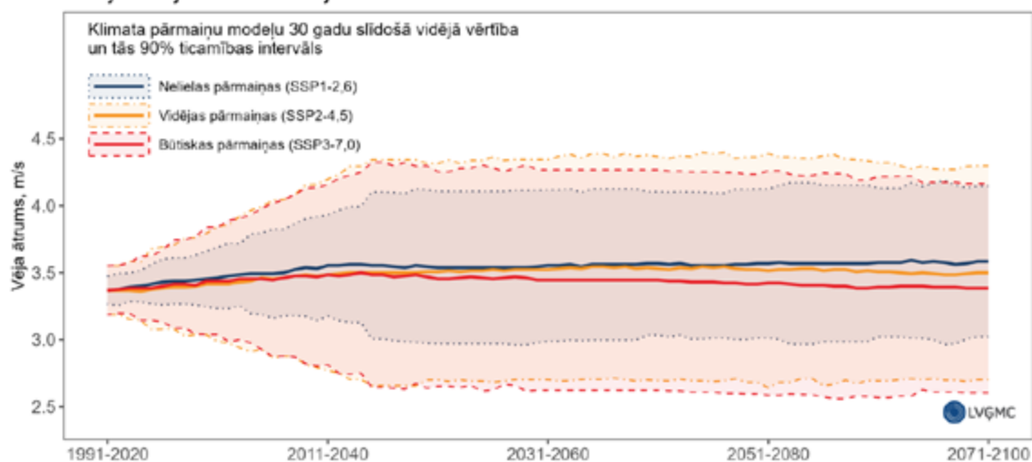
38. attēls Klimata pārmaiņu modeļu prognozētās Latvijas vidējās vēja ātruma 30 gadu slīdošās vidējās vērtības un to 90% ticamības intervāls līdz 21. gadsimta beigām
