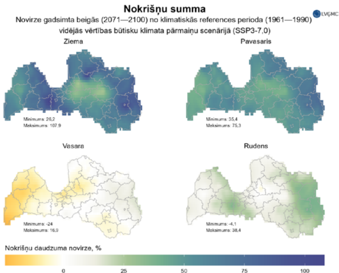
28. attēls Nokrišņu daudzuma izmaiņas ziemā, pavasarī, vasarā un rudenī, salīdzinot klimata pārmaiņu modeļu prognozētās 2071. līdz 2100. gada vērtības (SSP3-7,0) ar klimatiskās referenču periodā (1961.–1990. gads) novērotajām vērtībām
