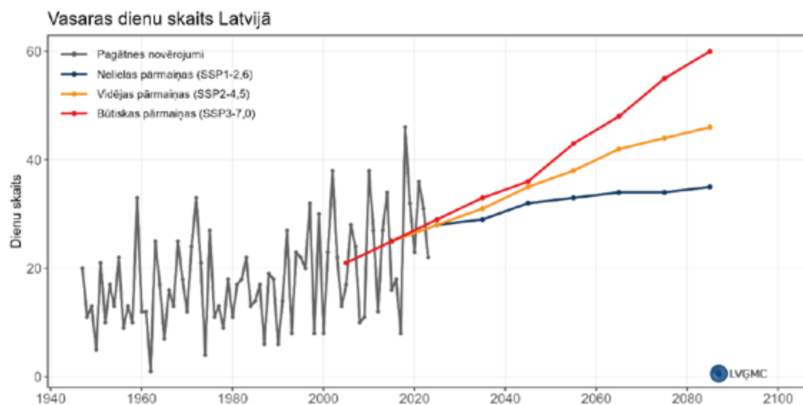
20. attēls Vidējais vasaras dienu skaits Latvijā, kas aprēķināts no meteoroloģisko novērojumu staciju datiem, kā arī nākotnes klimata pārmaiņu modeļu scenārijiem (SSP1-2,6; SSP2-4,5; SSP3-7,0)
