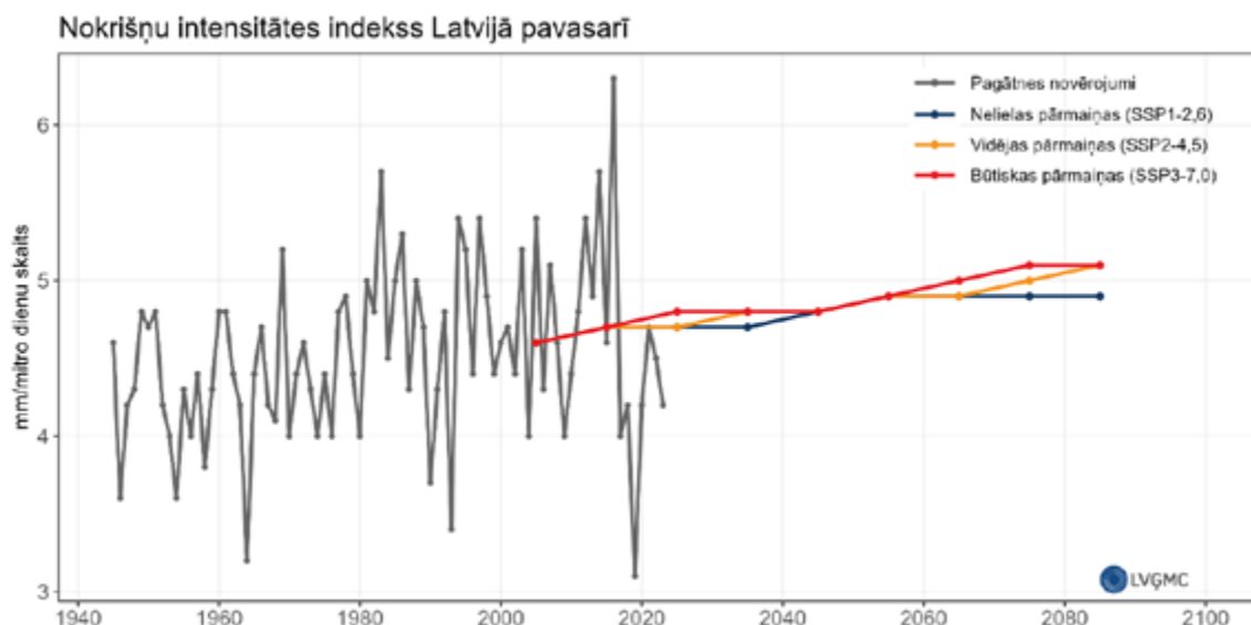
31. attēls Nokrišņu intensitātes indekss Latvijā pavasarī kopš 1945. gada (novērojumu dati) līdz 2100. gadam (klimata pārmaiņu modeļu scenāriju SSP1 2,6; SSP2-4,5 un SSP3-7,0 dati)
