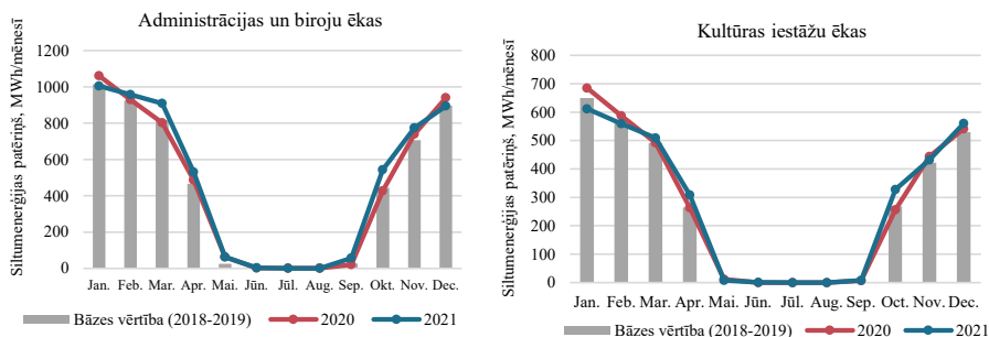
3.19. att. Siltumenerģijas patēriņš ar klimata korekciju, administrācijas un ofisu ēkās, un kultūras iestāžu ēkās, MWh/mēnesī.
