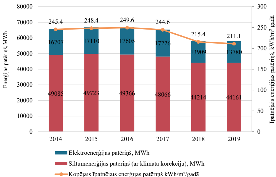
3.10. att. Kopējais enerģijas patēriņš 123 Daugavpils pašvaldības ēkās (2014 un 2015. gadā tikai daļēji vēsturiskie dati bija pieejami, tāpēc faktiskais enerģijas patēriņš bija augstāks).
