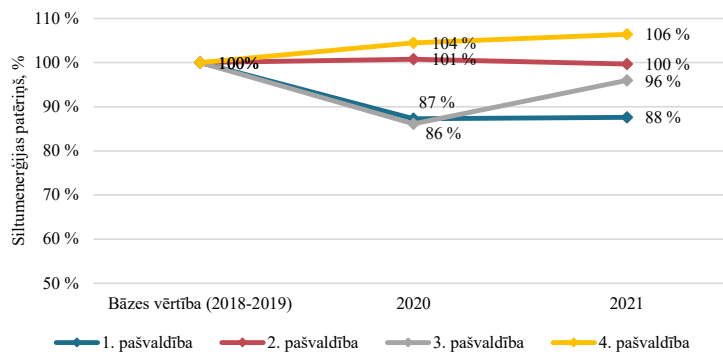
3.15. att. Apkures enerģijas patēriņa novirzes četrās pašvaldībās, salīdzinot ar bāzes scenāriju (2018-2019), %.
