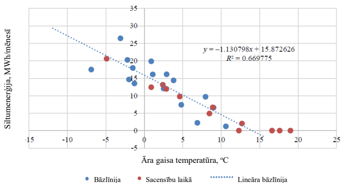
2.5. att. Piemērs siltumenerģijas bāzlinijas vērtības noteikšanai
