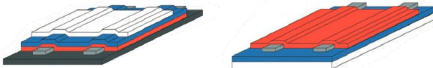
7. att. Organiskā lauka efekta tranzistoru shematisks atspoguļojums ar aizvara elektrodu virspusē (pa kreisi) un apakšā (pa labi). Polimēra substrāts (melns), izteces un noteces elektrodi (pelēki), organisks pusvadītājs (oranžs), izolators (zils), aizvara elektrods (balts). 83
