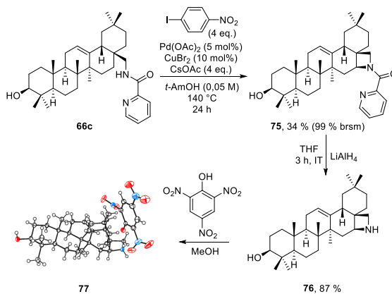
21. shēma. Azetidīna 76 veidošanās no pikolināmīda 66c .
