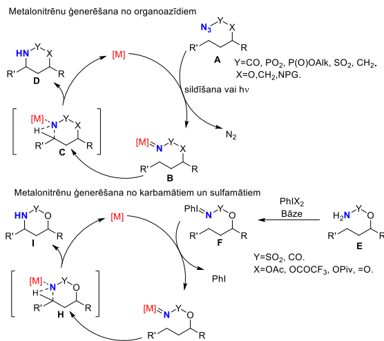
12. shēma. Metalonitrēnu ģenerēšanas mehānismi un sekojoša iespējamās C-H saitē.
