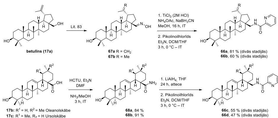
16. shēma. Pikolīnamīdu 66a-d sintēze.
