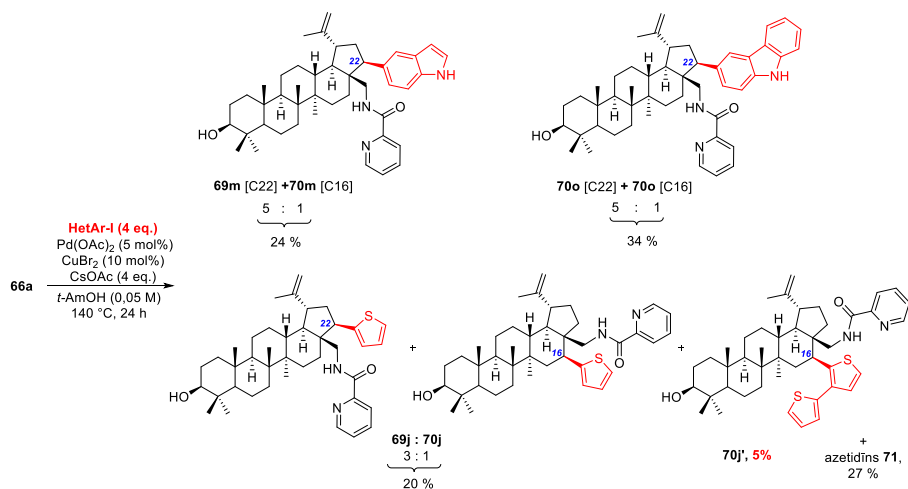
18. shēma. Pikolīnamīda 66a C( sp^3 )-H heteroarilēšana.
