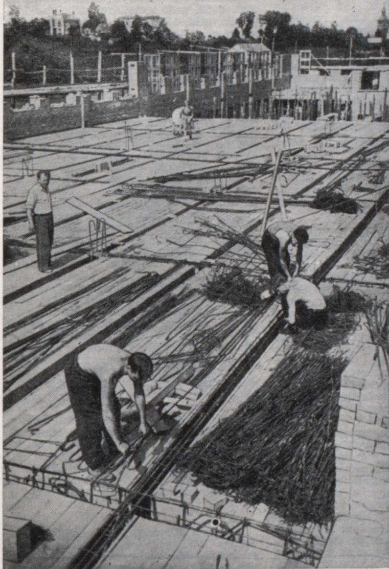
Sprāgi rit mēbeļu fabrikas celtniecības darbi. Attēlā: dzelzs stiegrājumu montaža jaunbūvē.
