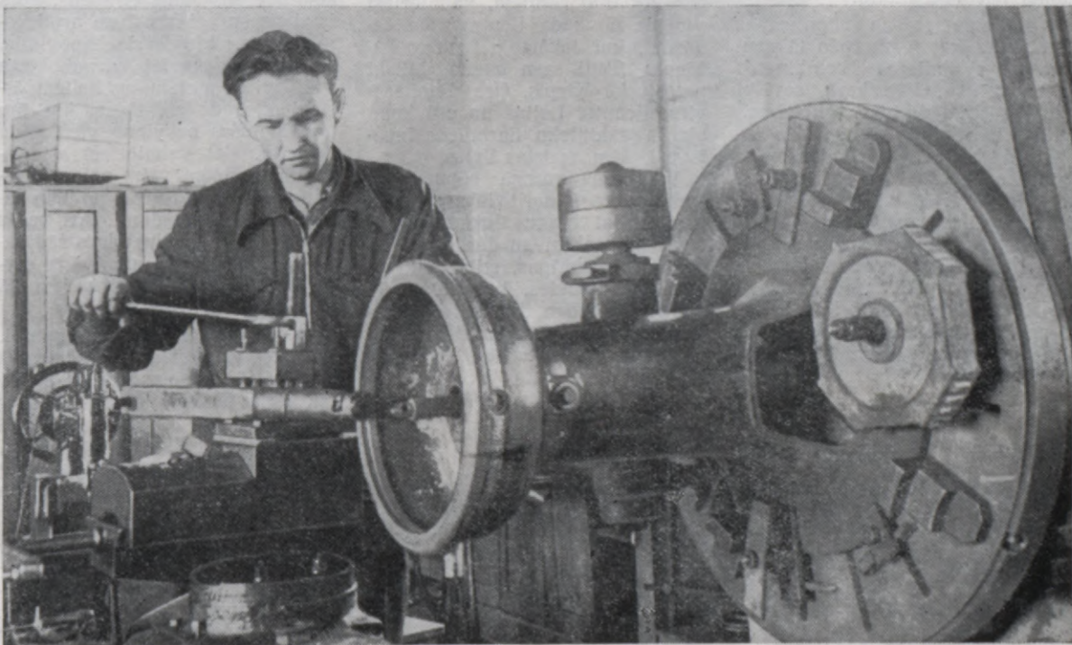
Rūpniecības kombināta labākais virpoļājs L. Nigals darbā.
