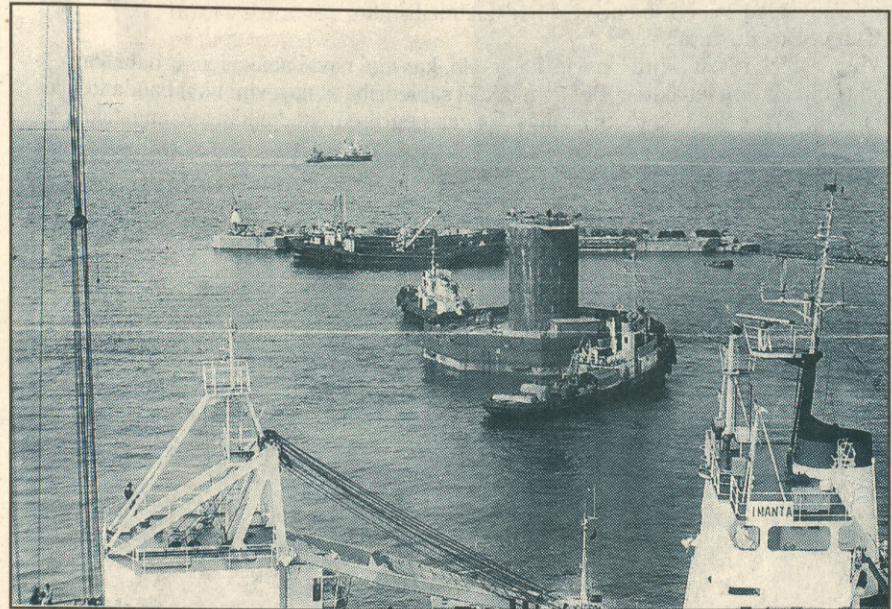
Irbes bākas būvdarbi 1985.gadā
