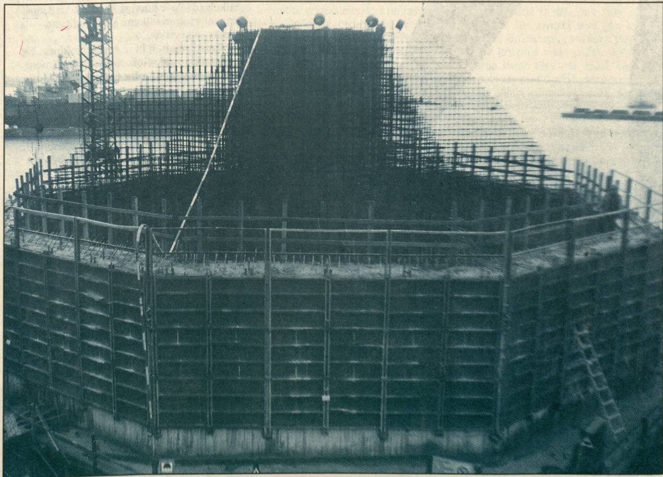
Bākas dzelzsbetona pamatu būvēja Tallinā. Foto — Jānis Trops un no A.Neilanda personiskā arhīva
