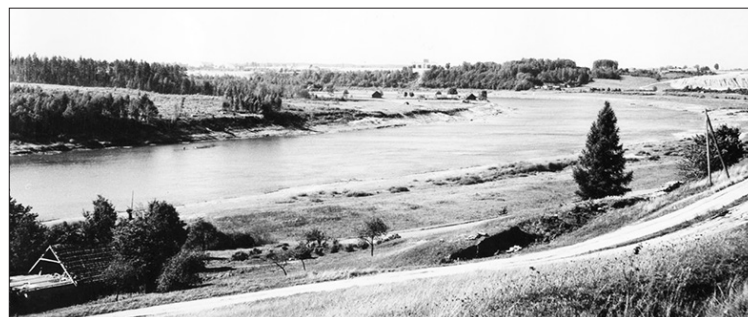
Aizkraukle. Samēnu līcis. Pļaviņu HES būvniecības laikā. Nākošā ūdenskrātuves applūdināšanas sākumā. Skats no labā krasta. 1963. g.
